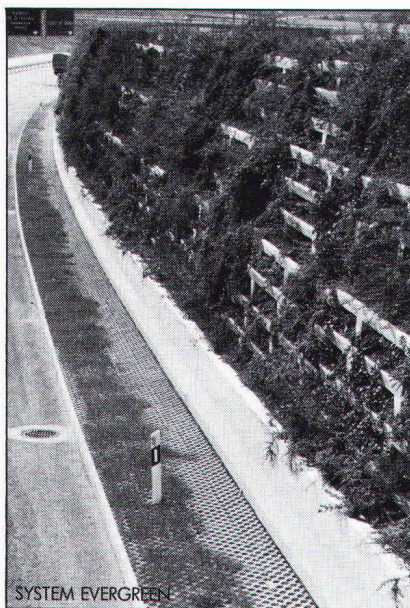
Bepflanzte Raumgitterwand
