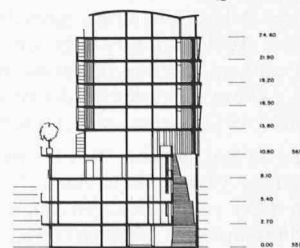
2. Obergeschoss Querschnitt
