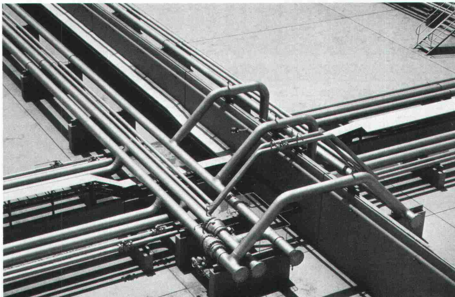
Brennstoff-Verteilnetz im Tankfeld
