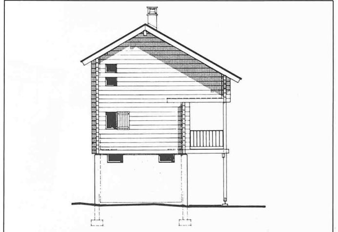
Reconversion d'un grenier en habitation de vacances, Evolène 1968-1969 Vincent Mangeat, Nyon
