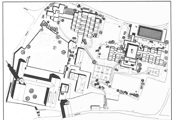
Collège, Brigue 1961-1978 Groupe 61, Lausanne
