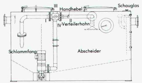
Fettabscheider-Anlage LIPURAT-Standard Geruchlos arbeitende Anlage aus Stahlblech mit automatischer Entleerungs- und Spüleinrichtung.
