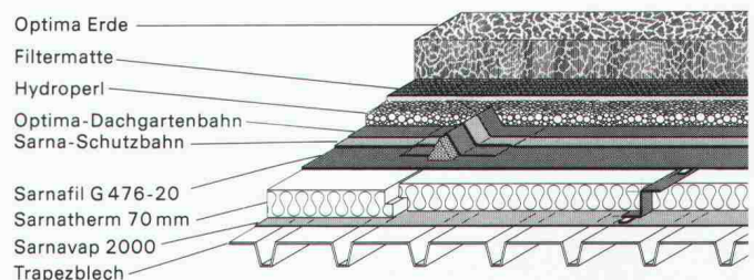
Schichtaufbau des begrüneten Jumbo-Flachdaches mit optima-System.
