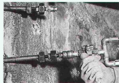
Flankierende Massnahmen: Injektions-Abdichtungen von Rissen und Rohrdurchführungen am Rohbau.
