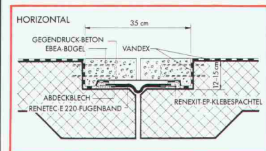
Renesco-Abdichtungen von Dilationsfugen im Grundwasserbereich.
