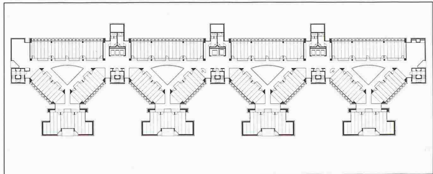
Grundrisschema Bürogeschoss
