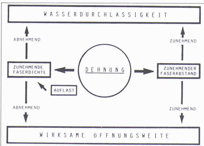
Bild 1. Filtertechnische Auswirkungen der Dehnung eines Geotextils (Saathoff)
