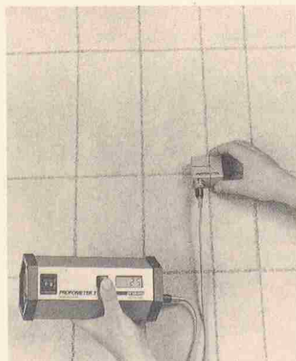
Bewehrungssucher Profometer 3
