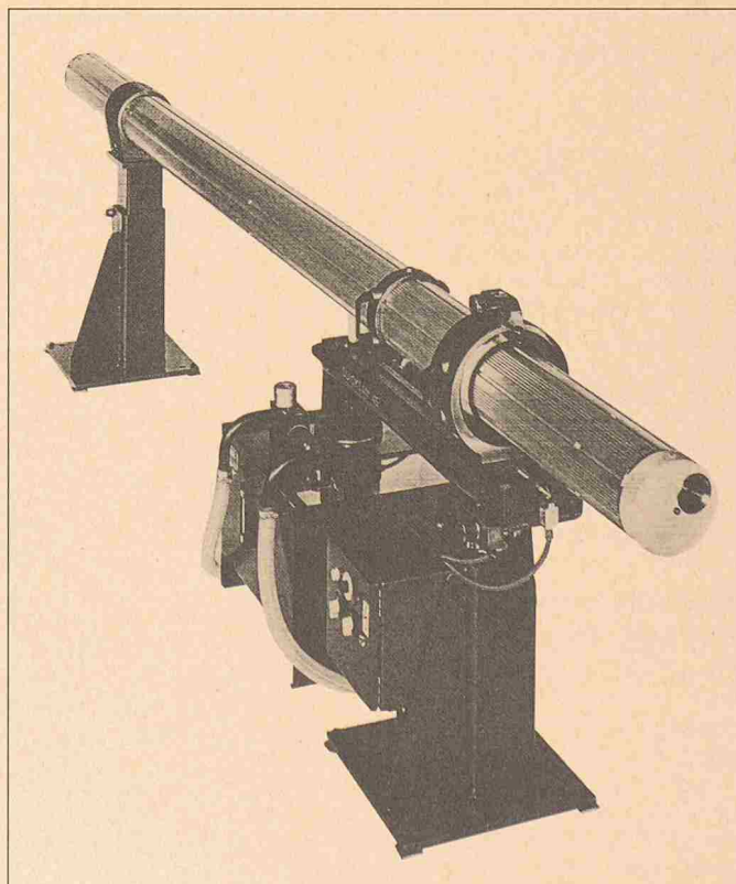
Bild 2. Ansicht der Stangenzuführung «Quicksam-45» für Drehautomaten (Sameca SA, Lamboing)
