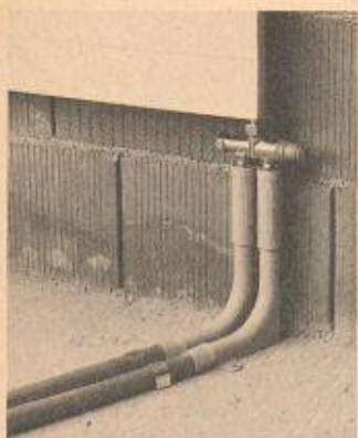
Das neue Heizkörper-Anschlussystem von Gunzenhauser
