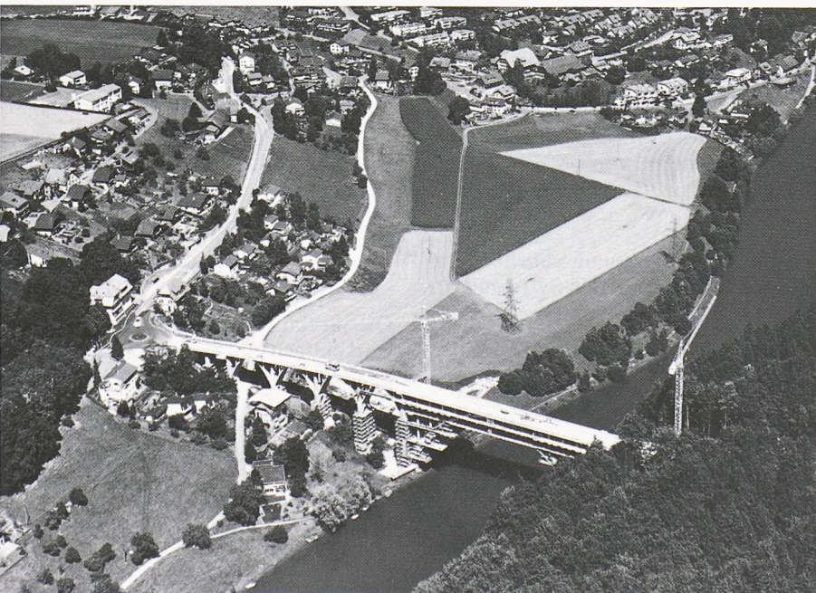
Die Baustelle Halenbrücke aus der Vogelperspektive. Unter anderem mussten die vier Bogen der Vorbrücke (links) und die gesamte Fahrbahnplatte ersetzt werden (Bild: Comet)
