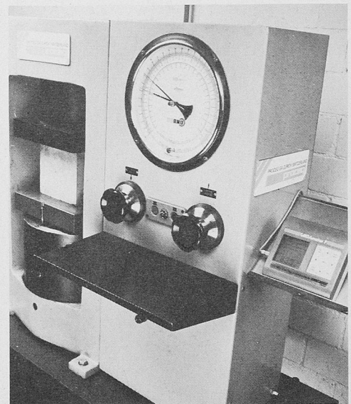
Durch den Anschluss eines Wiggameter-Anzeigergerätes (rechts) können ältere Druckprüfmaschinen hochgerüstet werden
