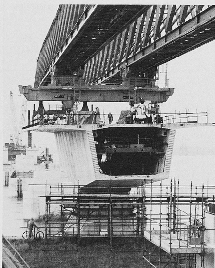
Eine der Brückentafelteile aus Stahlbeton wird durch einen Portalkran in die gewünschte Lage gebracht
