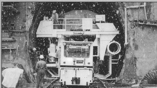
Konsolidierungsbereich am Nordportal des Vereinatunnels
