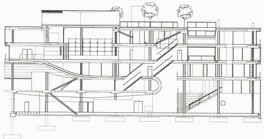
Villa VPRO, Hilversum, 1993–97. Architekten MVRDV, Rotterdam. Schnitt
