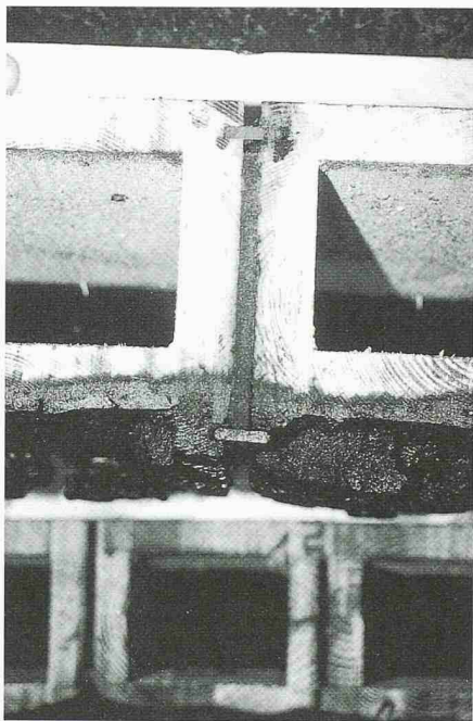
Ausschnitt einer Elementdecke nach dem Brandversuch vom Oktober 1998. Die ursprüngliche Holzstärke lässt sich anhand der verkohlten Stellen noch abschätzen
