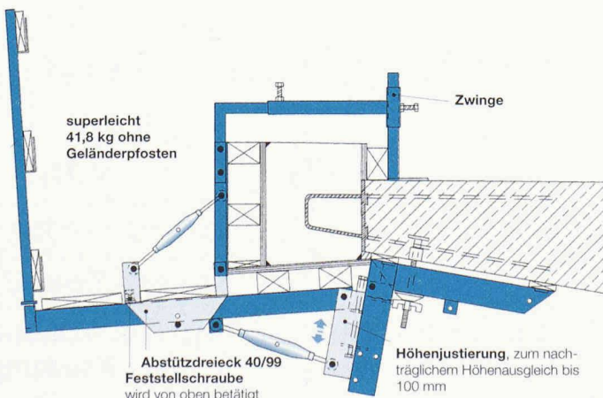
Quick-Kappenriegel Typ 98 mit Höhenjustierung und Abstützdreieck 40/99
