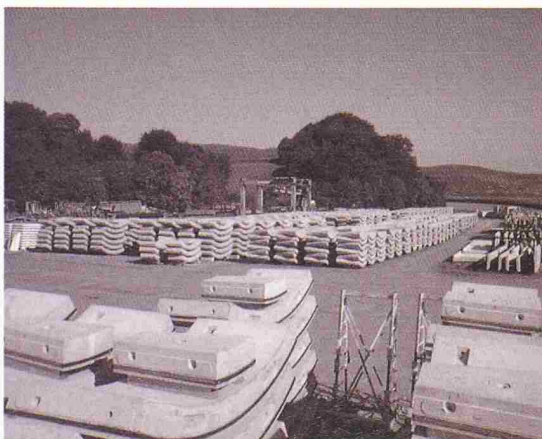
Flughafen Zürich / Tübbings für das Personentransportsystem
