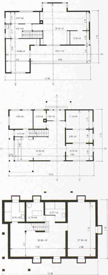
Pläne von oben nach unten: Obergeschoss, NF 76 m 2 ; Erdgeschoss, NF 85 m 2 ; Untergeschoss, NF 79 m 2 . Das Kellergeschoss, das an der Saffa-Ausstellung 1928 nicht existierte und erst in Aarau neu erstellt wurde, wird beim Wiederaufbau neu gebaut werden (Bilder: aus der Dokumentation des Vereins proSAFFAhaus, Küsnacht)
