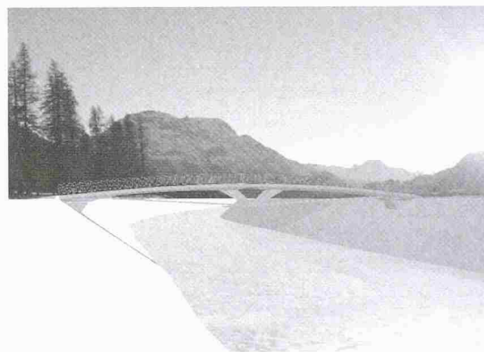
1. Rang Flazbrücken Samedan: Perspektive und Längsschnitt (Mst. 1:500) für den Standort Gravatscha von Ingegneri Pedrazzini und Baserga Mozzetti architetti. Für die ständigen Lasten funktioniert die Struktur als Bogen mit Zugbändern. Die Diagonalen verleihen der Fahrbahn die erforderliche Steifigkeit zur Aufnahme der variablen Lasten. Material: Beton, Zugbänder und Diagonalen vorgespannt (Bilder Projektverfasser)
