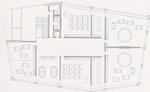
1. Obergeschoss des neuen Primarschulgebäudes (1. Rang, Businger + Odermatt)
