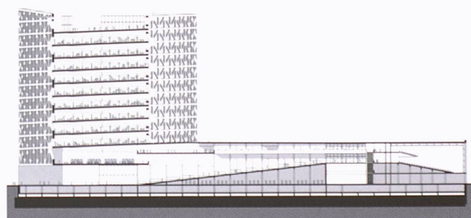
Coupe sur l'ensemble du bâtiment
