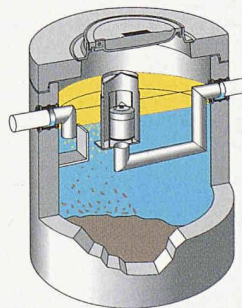
Leichtflüssigkeitsabscheider
