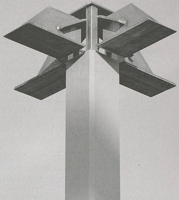
Stützenkopfverstärkung T-WALM ®
