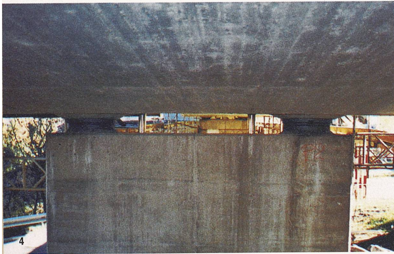
3 Einbau eines neuen Topfgleitlagers im talseitigen Widerlager WL1
