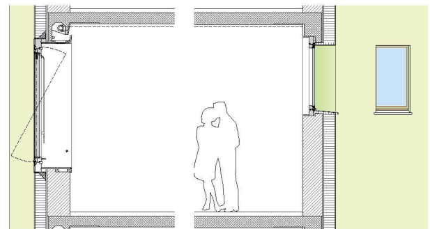
01+02 «Foulard»: Das Spiel der neuen Kippfenster belebt die sanierte Südfassade, im Norden wird die Wärmedämmung verstärkt (Bilder: Verfassende)
