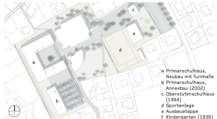
01+02 «Erlenstrauss»: Der Neubau fasst dreiseitig den Pausenhof, südlich vermittelt die Pausenhalle zum Annexbau (Bilder: Verfassende)
