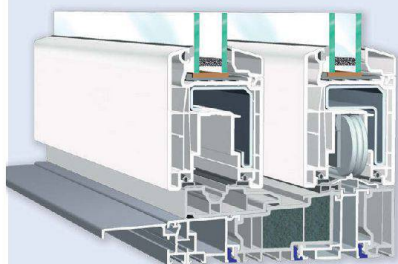
VEKASLIDE Hebe-Schiebetür
