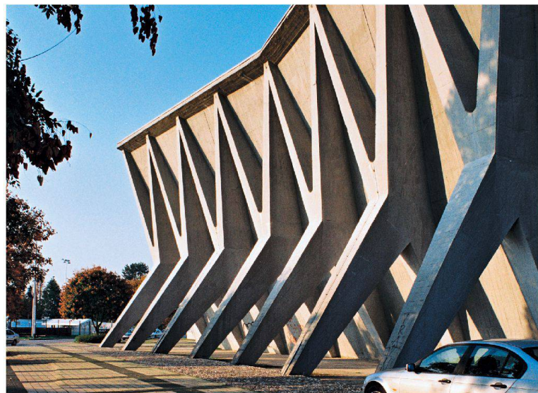
Pavillon der Zagreber Messe (1958) von Ivan Vitić: Kräftige Stützen halten das hängende Dach.
