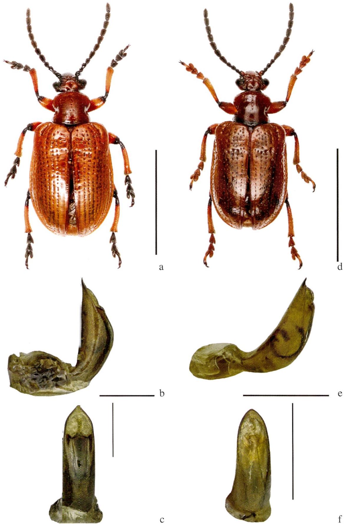
Abb.1: Lilioceris schneideri von Hemmental SH. — Männchen 1, a-c und Männchen 2, d-f. — Habitus, a und d, Skala = 5 mm; — Aedeagus lateral, b und e, Skala = 1 mm; — Aedeagus dorsal, c und f, Skala = 1 mm.
