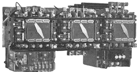
Sterndreieckschütze MSSp 40
