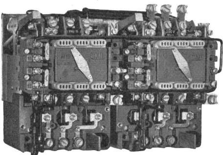
Polumschaltshütze MWp 15/25 für Motoren mit 2 getrennten Wicklungen
