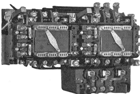
Drehrichtungsumschaltschütze MDp 15/25
