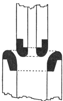
HOCHSPANNUNGS- LEISTUNGSSCHALTER
