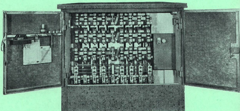
* FUCHS-Kabelverteilkabine II
