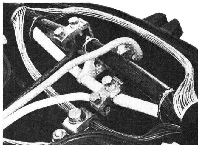
T-Abzweigungsmuffe mit Ceanderkabel, Leiter nicht abisoliert
