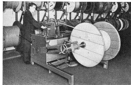
Type TR 125 Umtrommelmaschine lieferbar für Kabel bis 80 mm \phi
