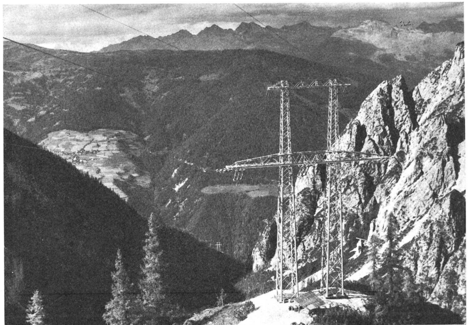
Fig. 3 220-kV-Kupplungsleitung Österreich—Italien
