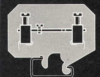
Durchgangsklemme mit einseitiger Querverbindung
