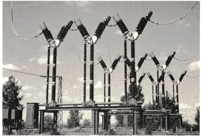
Fig. 5 Ölarmter Hochspannungsschalter 420 kV, Nennauschaltstrom 50 kA, Nennstrom 3150 A Fabrikat ASEA, Schweden
