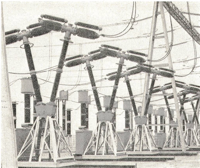
Fig. 6 SF 6 -Eindruck-Hochspannungsschalter 420 kV, Nennauschaltstrom 40 kA, Nennstrom 2000 A Fabrikat Delle-Alsthom, Frankreich
