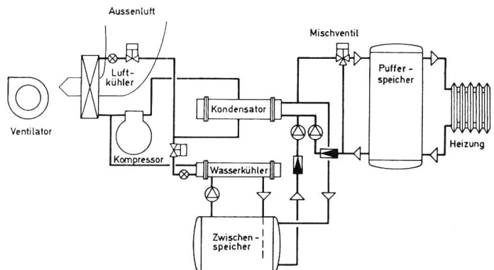
Prinzipschema der zweistufigen Aerocal-Wärmepumpe
