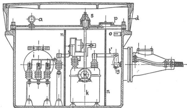
Fig. 2 Hochspannungskabelkasten, 1913 (Voigt & Häffner) [A1]
