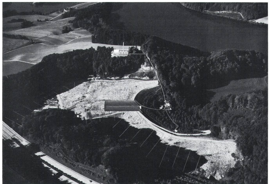
Figur 1 Das grösste schweizerische Deponiegas-Kraftwerk in Teuftal
