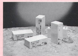
Miniatur-Starkstrom-Relais
