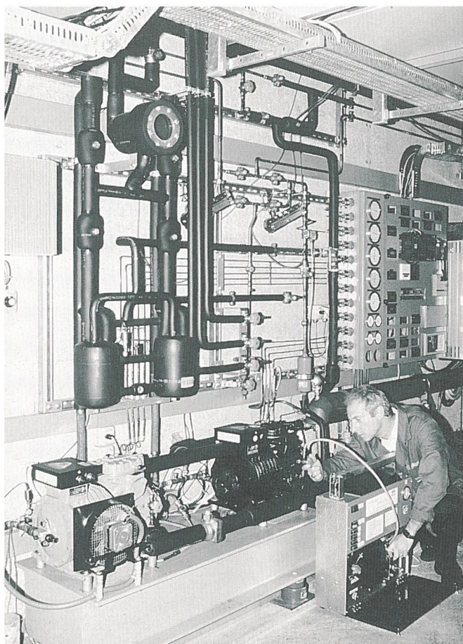
Bild 2 Forschungsanlage EICH: Nach Betriebsversuchen an der Drehzahlgrenze wird das Kältemittel aus den Verdichtern abgesaugt, um die durch das Abweichen von der Normdrehzahl gefährdeten Bauteile ihrer Zylinderköpfe zu inspizieren. Rechts am Bildrand ein Wandschrank mit Überwachungsinstrumenten (Photo Eggenberger)
