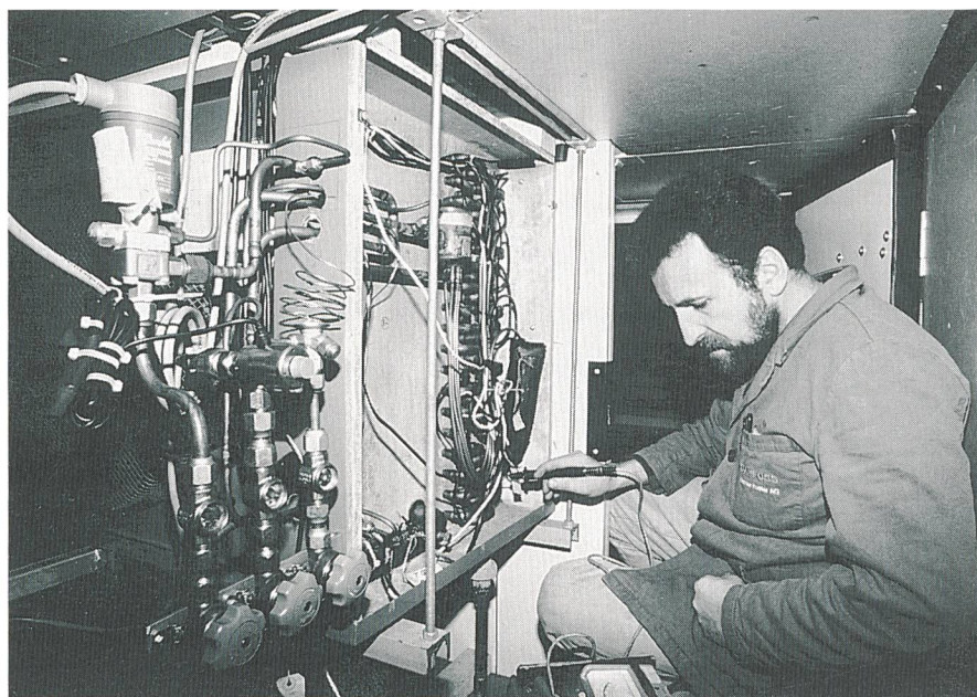
Bild 3 Forschungsanlage EICH: Vertrauen in die computerisierte Messung ist gut, Kontrolle mit Handmessung besser – hier die Regelungsstabilität der Kältemittelüberhitzung. Diese Regelung, für die drei Varianten untersucht werden, ist entscheidend für den Wirkungsgrad einer Wärmepumpen-Anlage (Photo Eggenberger)
