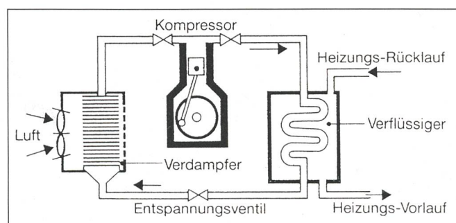
Bild 1 Prinzipschema einer Wärmepumpe
