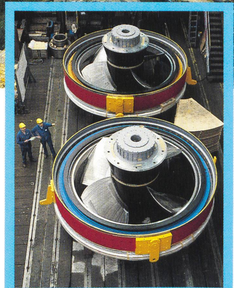
Die Straflo-Lauffräder Nr.1 für Augst und Wyhlen sind transportbereit. Vor Ort werden die von ABB gefertigten Generatorpole auf dem Laufradkranz befestigt (Juni 1992).
