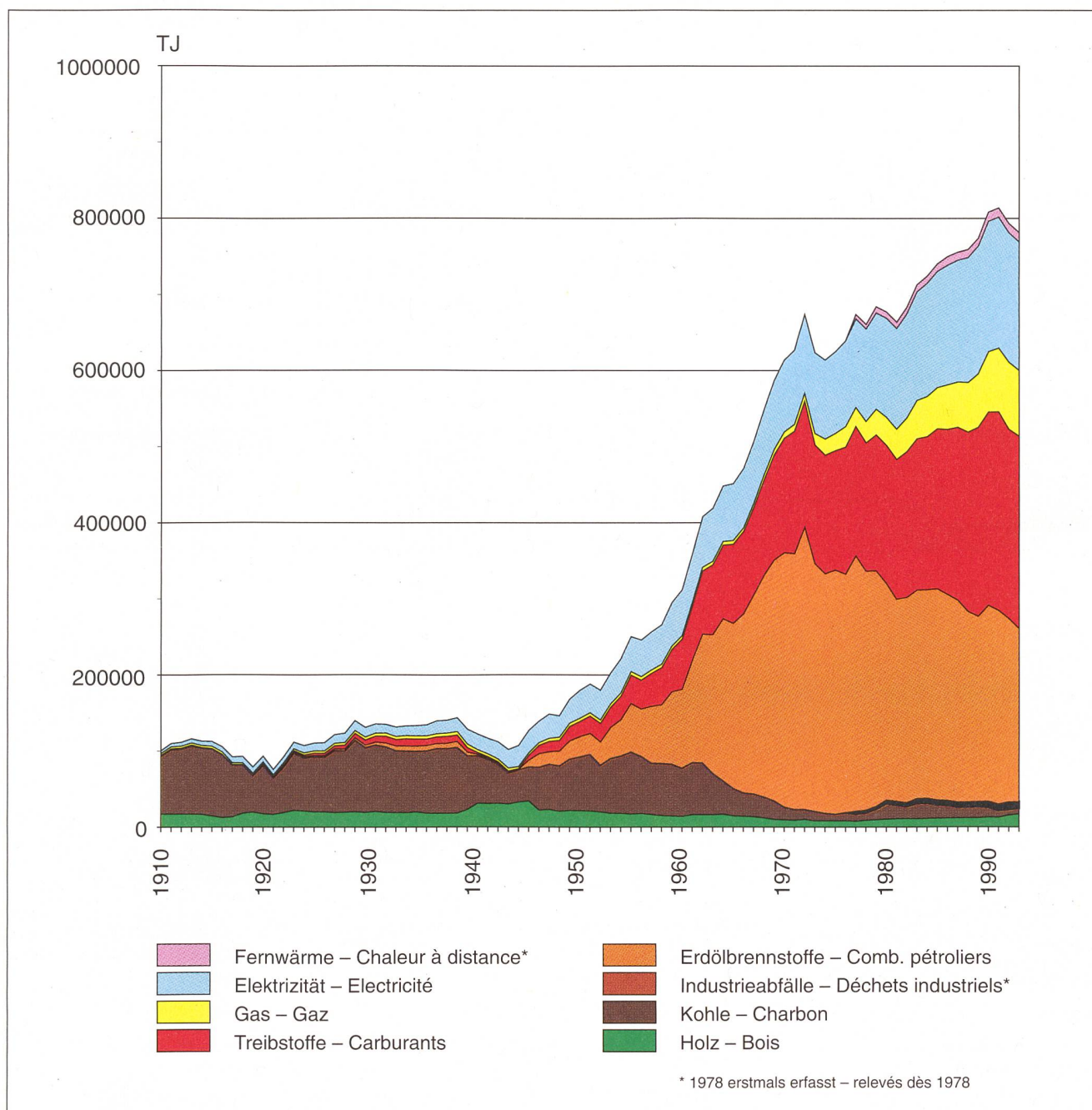
Fig. 1 Endenergieverbrauch 1910–1994 nach Energieträgern Consommation finale 1910–1994 selon les agents énergétiques
