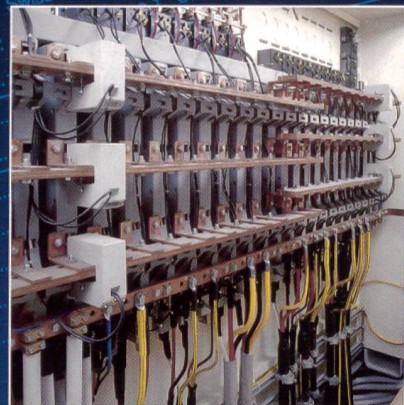
Schienensystem: flachliegend/horizontal
