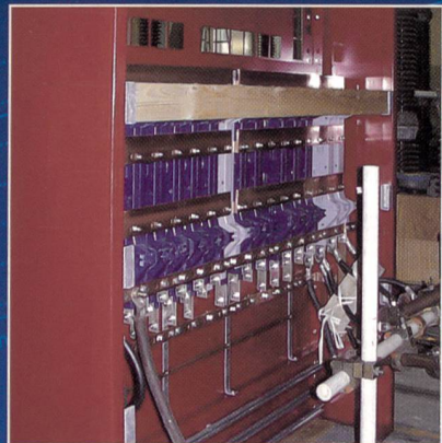
Schienensystem: hochstehend/vertikal
