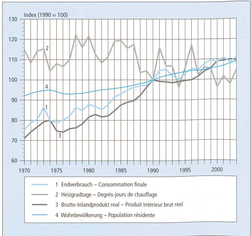
Fig. 14 Entwicklung energie-relevanter Größen im Vergleich zum Endverbrauch
