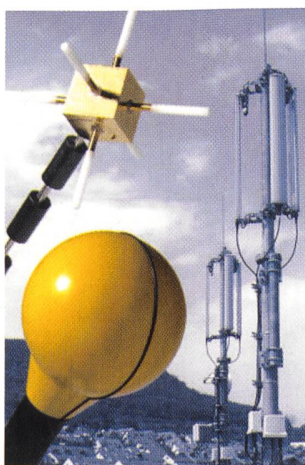
Die neue Sonde von Narda STS erfasst einen Frequenzbereich von 80 MHz bis 3 GHz
