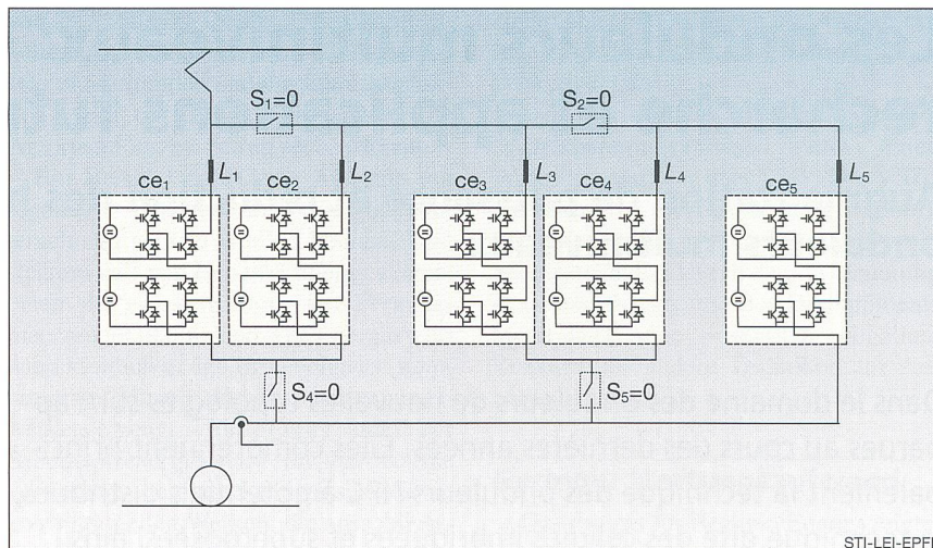
Figure 4 Convertisseur configurable pour locomotive multicourants
