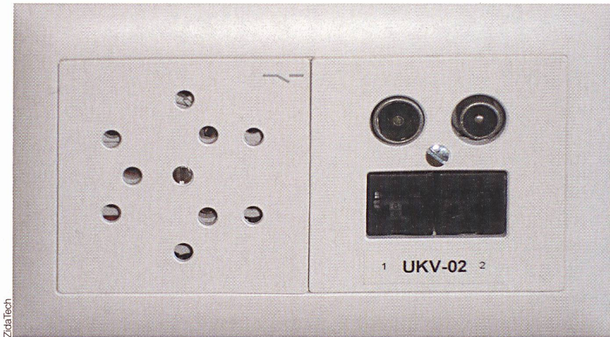
Bild 3 Kombinierte Steckdose mit RJ45 für EDV, Internet und Telefon sowie Koaxialanschlüsse für SAT und TV.
