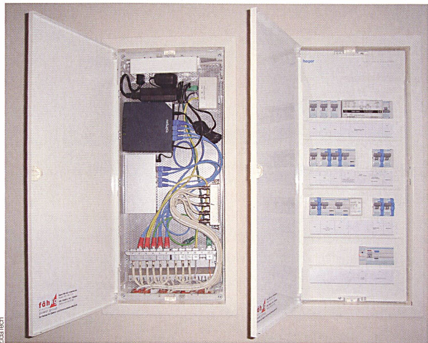
Bild 2 Neben dem Stromverteiler ist ein Medienverteiler platziert, mit Modems und Router.
