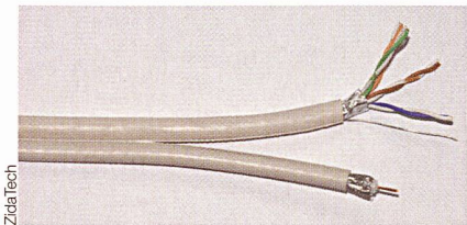
Bild 1 Systemkabel HomeWayPlus: Duokabel mit Kat.-5-Netzwerkabel und Koaxialkabel bis 2400 MHz.
